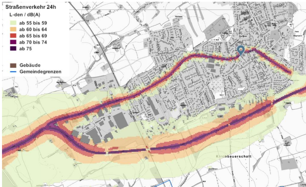
Abb. 01 – Umgebungslärm NRW – Lärmkarten 4. Runde 2022 Gemeinde Nordwalde
