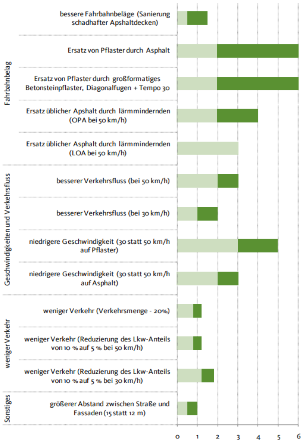
Abb. 10 Darstellung möglicher Lärminderungspotenziale in dB(A)
