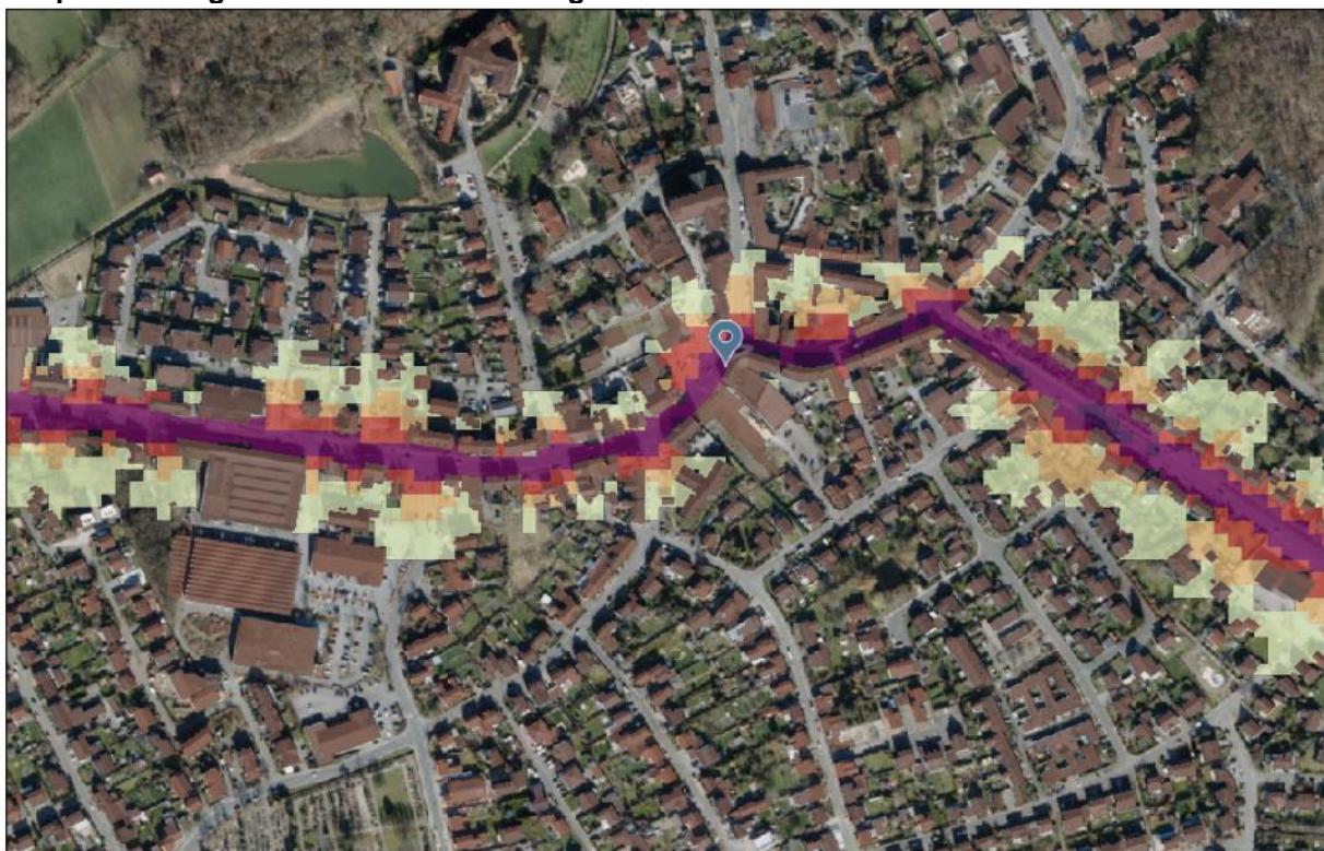
Abb.05 Lärmaktionsplan Stufe 4 – Gemeinde Nordwalde – Hauptkartierung Nordwalder Ortskern-Tag
